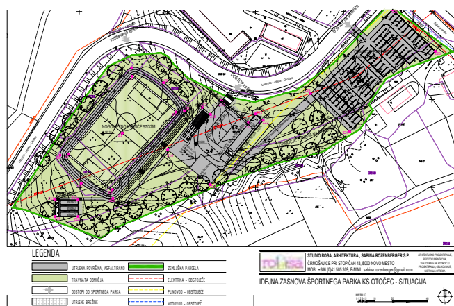
Idejna zasnova športno rekreacijskega parka Otočec.
