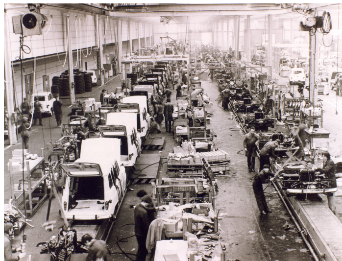
Montaža šasije katrce konec 70-ih let.
